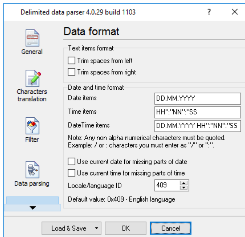
Data format
