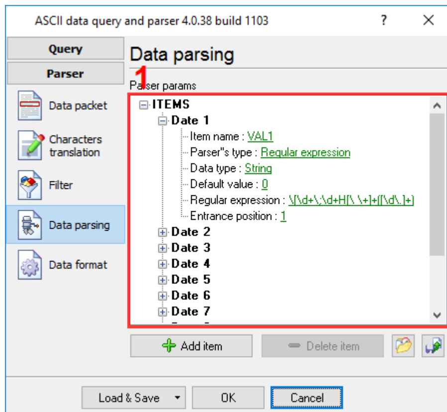
Fig.3.1. Parser variables
