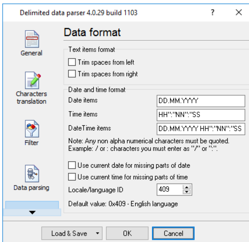
Data format
