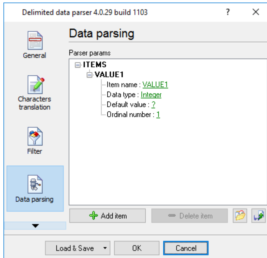
Fig.2. Data parsing
