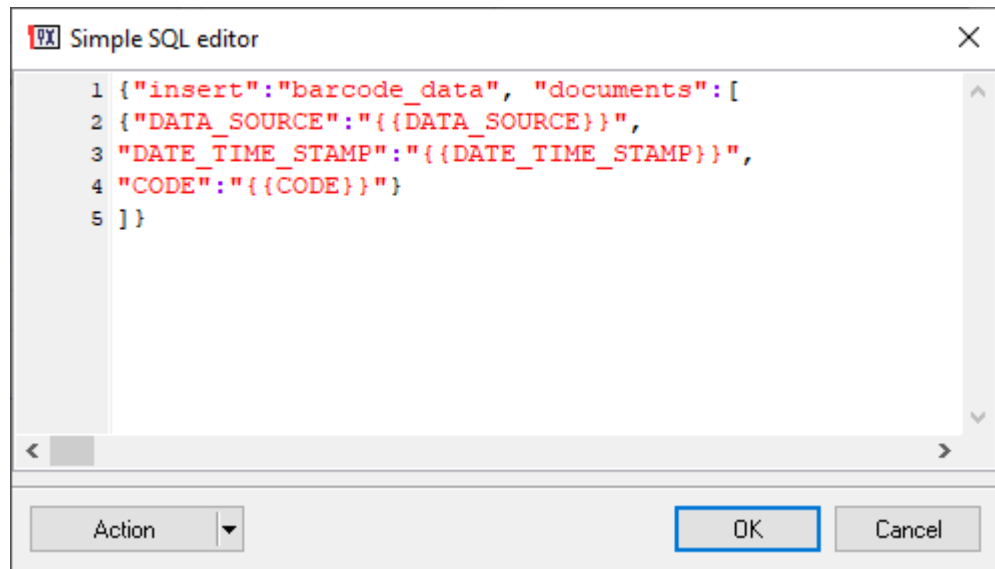
Fig. 8. Insert statement
