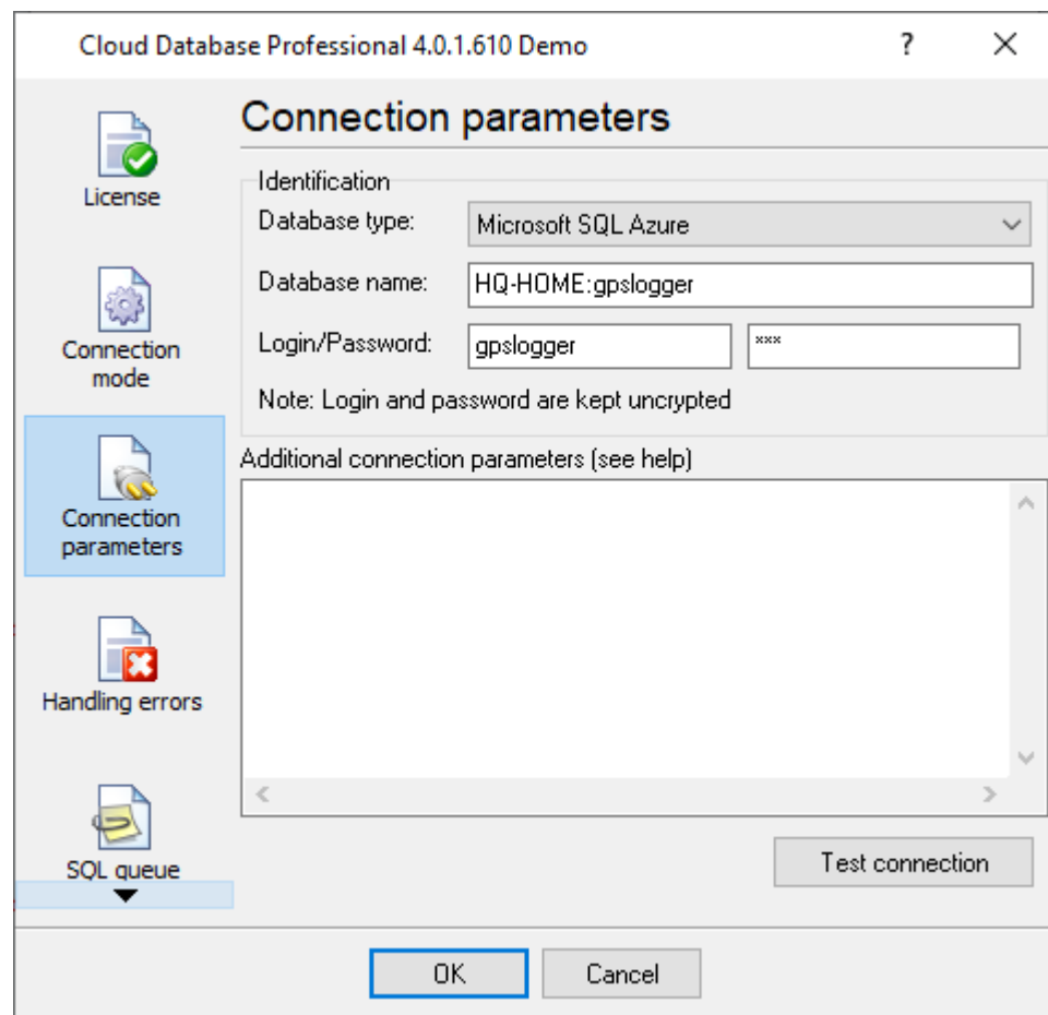
Fig. 2. Connection parameters
