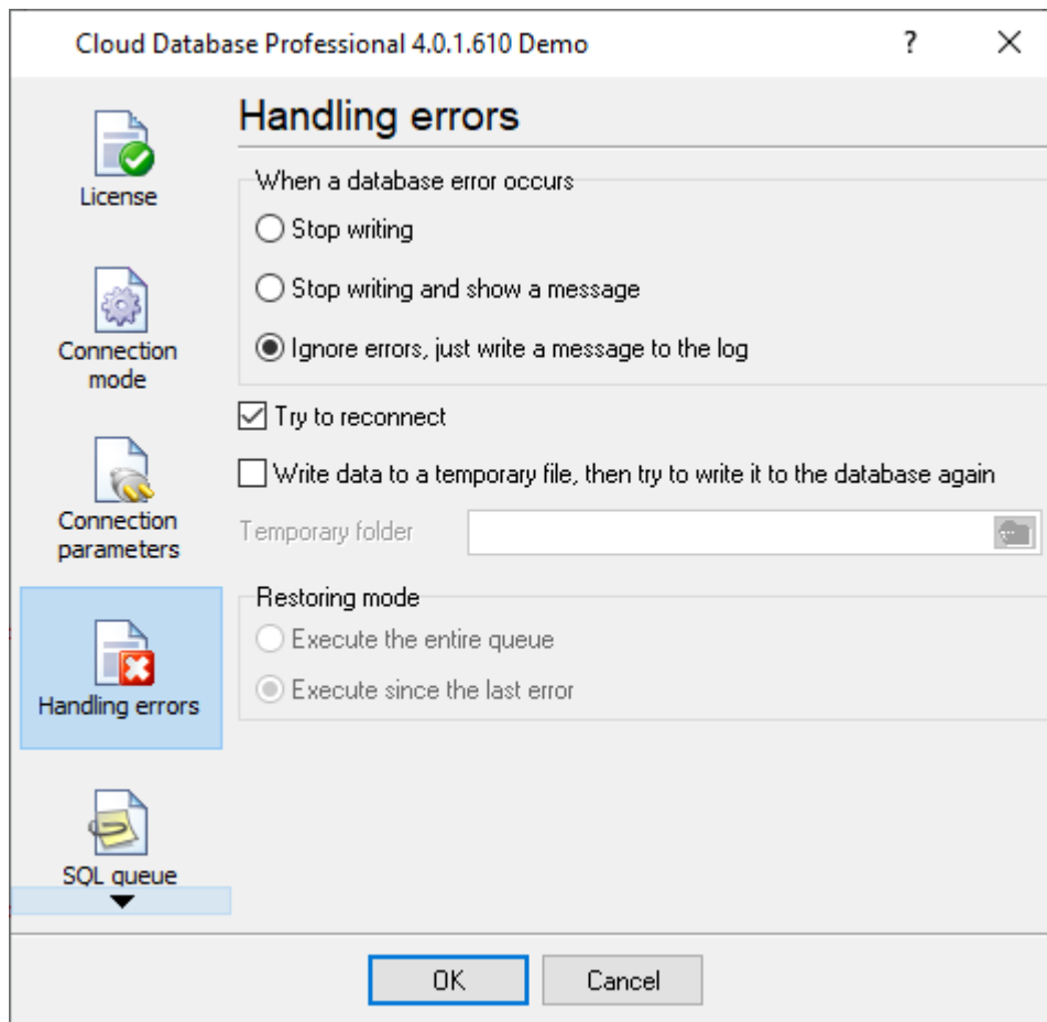
Fig. 9. Handling errors
