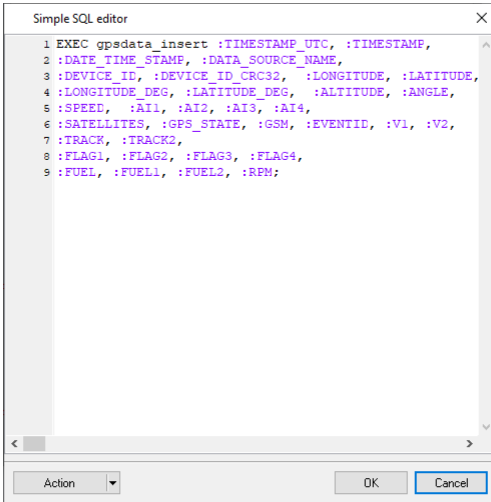
Fig. 12. SQL editor
