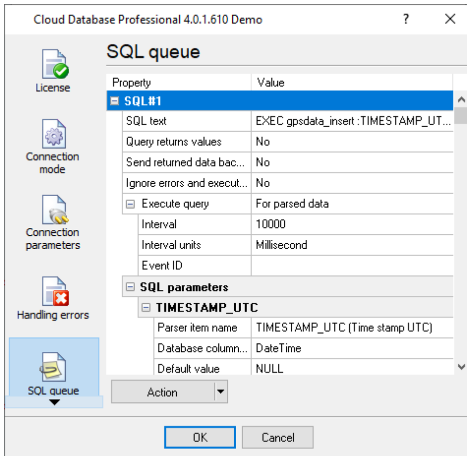
Fig. 10. SQL queue
