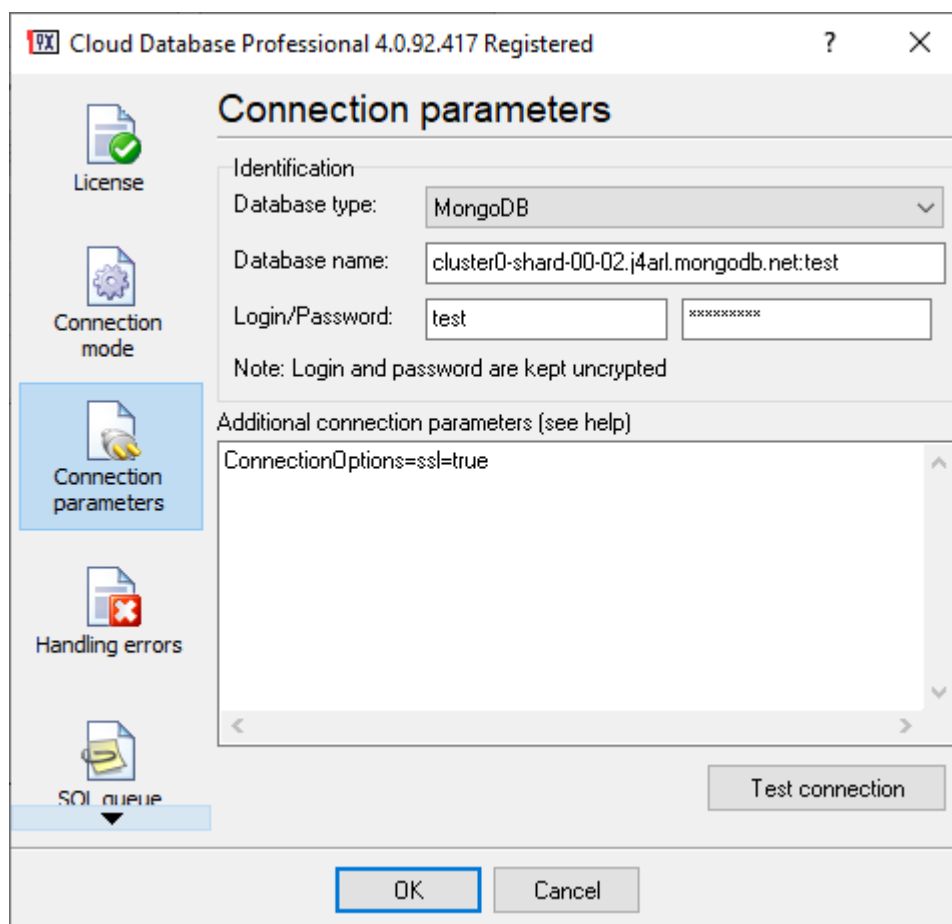
Fig. 7. Connection parameters
