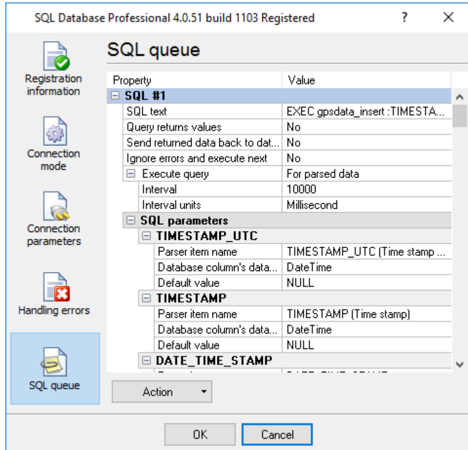
Fig. 5. A new SQL query
