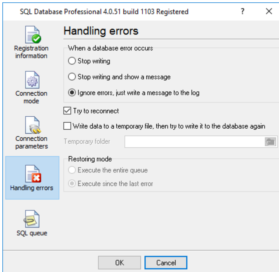
Fig. 3. Handling errors
