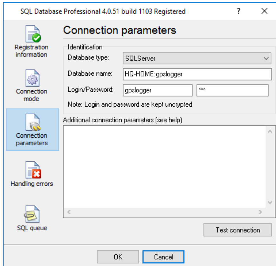
Fig. 2. Connection parameters
