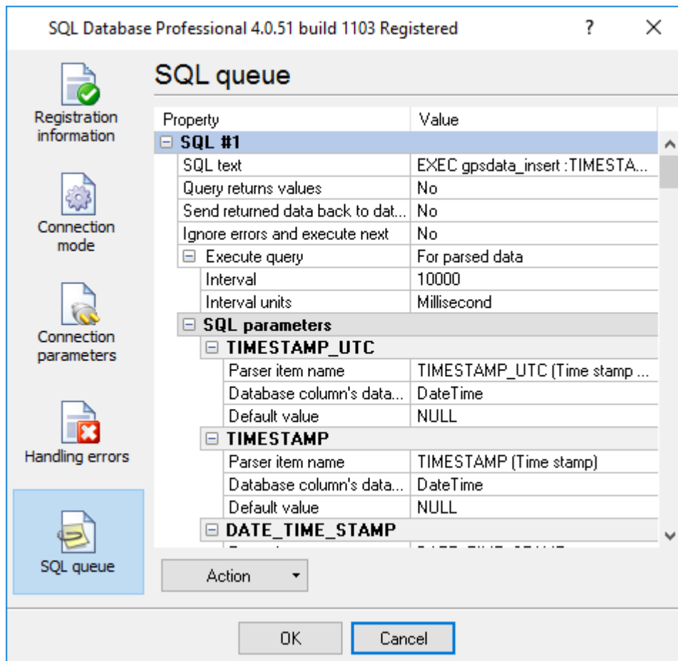
Fig. 4. SQL queue
